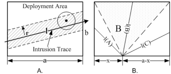
Fig. 21. Intrusion Model
