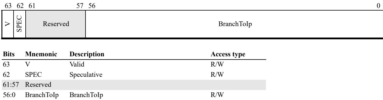
Figure 13-8. LastBranchStackToIp MSR
